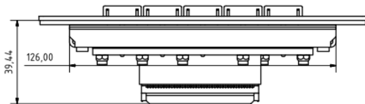
ANSICHT (VIEW)1 ( 1 : 1 )
